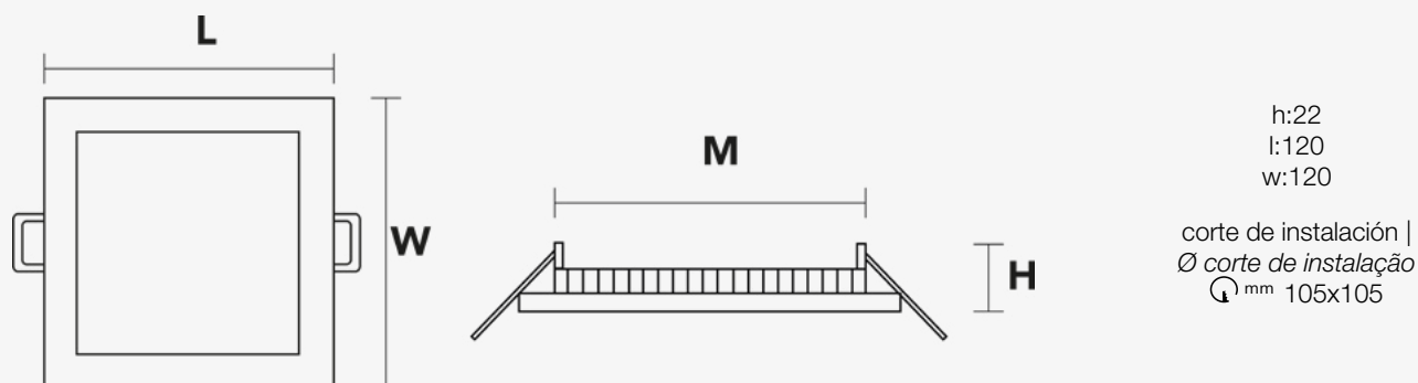
Esquema de Producto. Product line drawing
